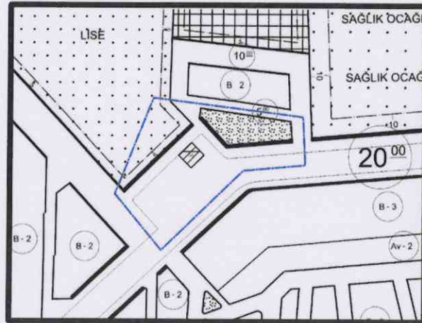
1/1.000 Ölçekli Mevcut Uygulama İmar Planı
