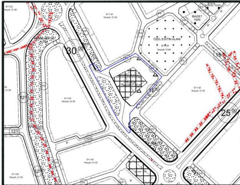
1/1000 Ölçekli Öneri Uygulama İmar Planı
