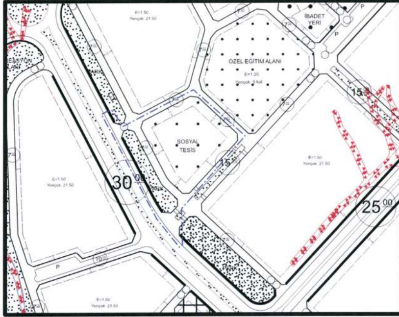
1/1000 Ölçekli Mevcut Uygulama İmar Planı
